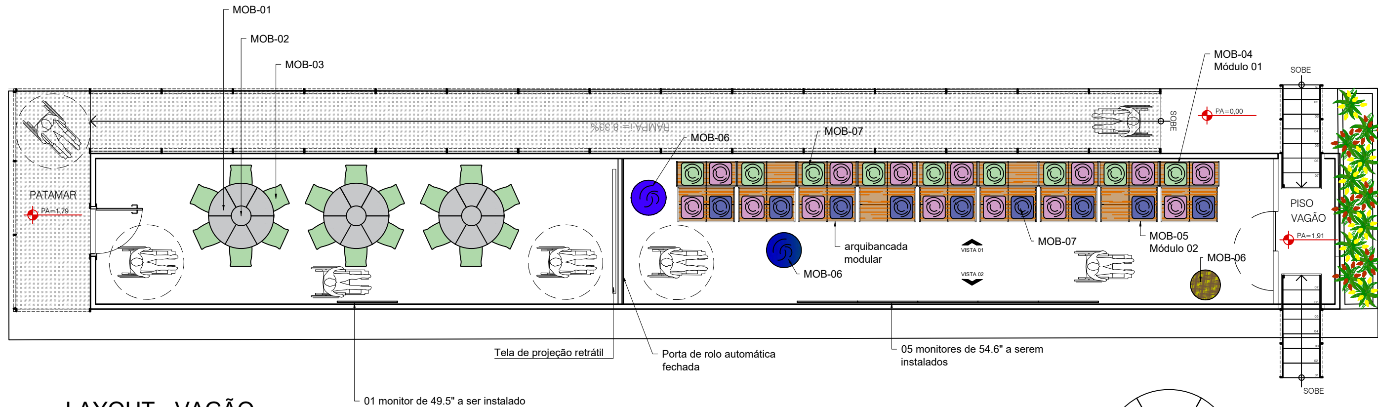
01 LAYOUT - VAGÃO ESC: 1/75
